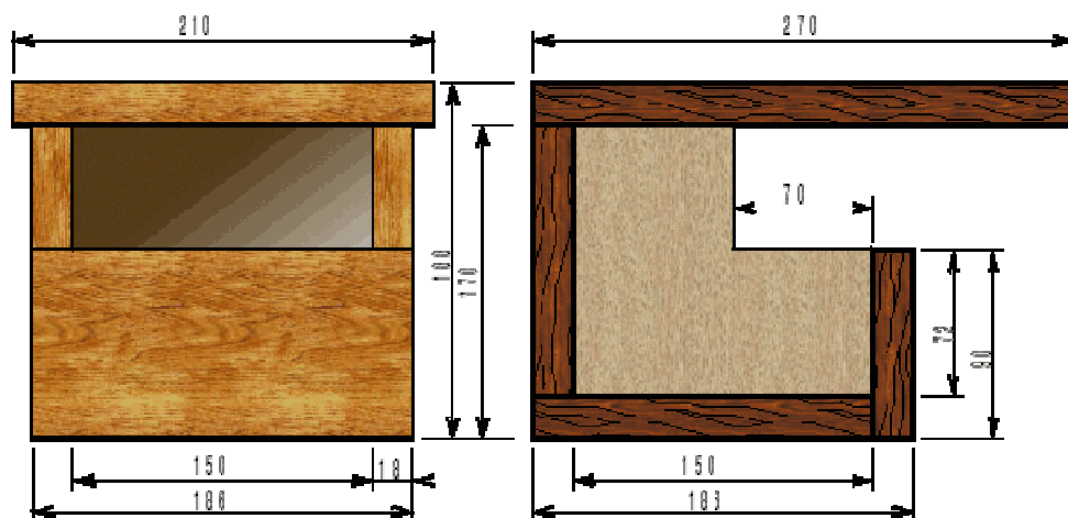
Figure 88 : Modèle de nichoir « semi-ouvert ».
