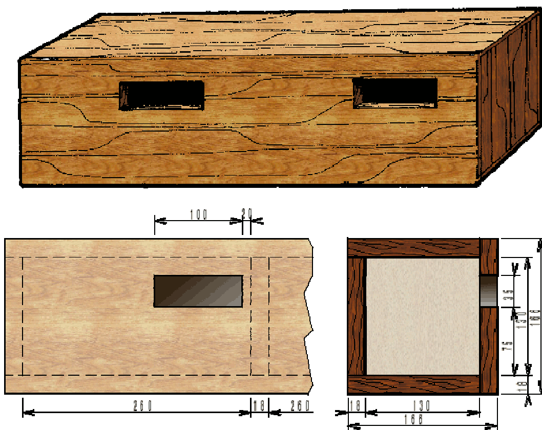
Figure 89 : Modèle de nichoir à Martinet noir.
