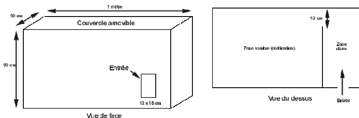
Figure 83 : Modèle de nichoir pour l'Effraie des clochers, GECNAL, 2006
