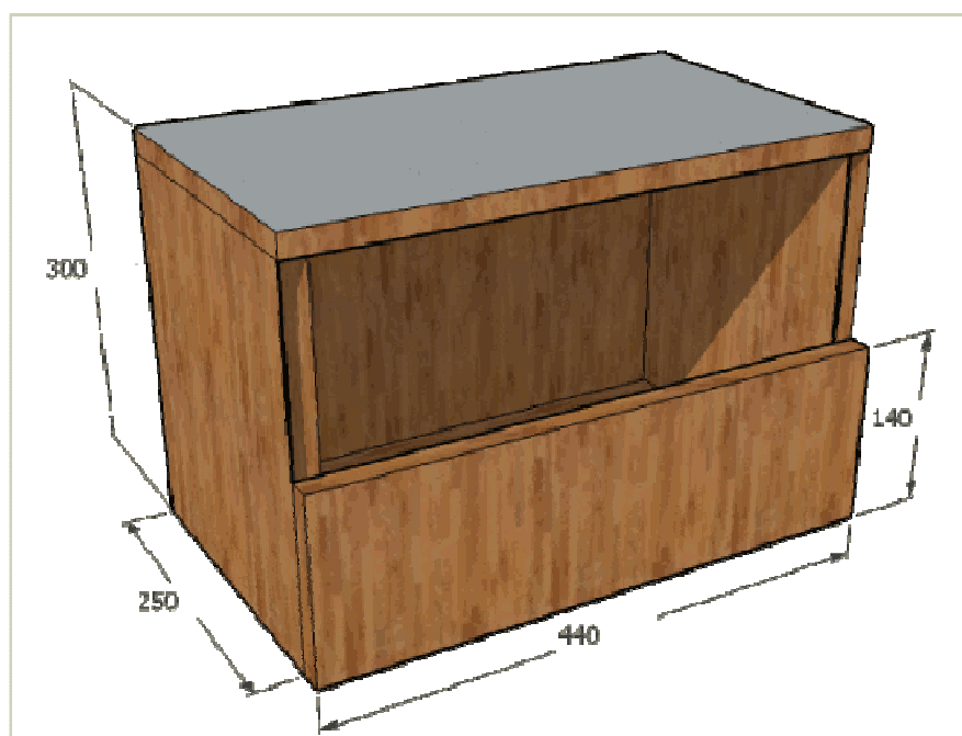
Figure 92 : Modèle de nichoir à Faucon crécerelle.
