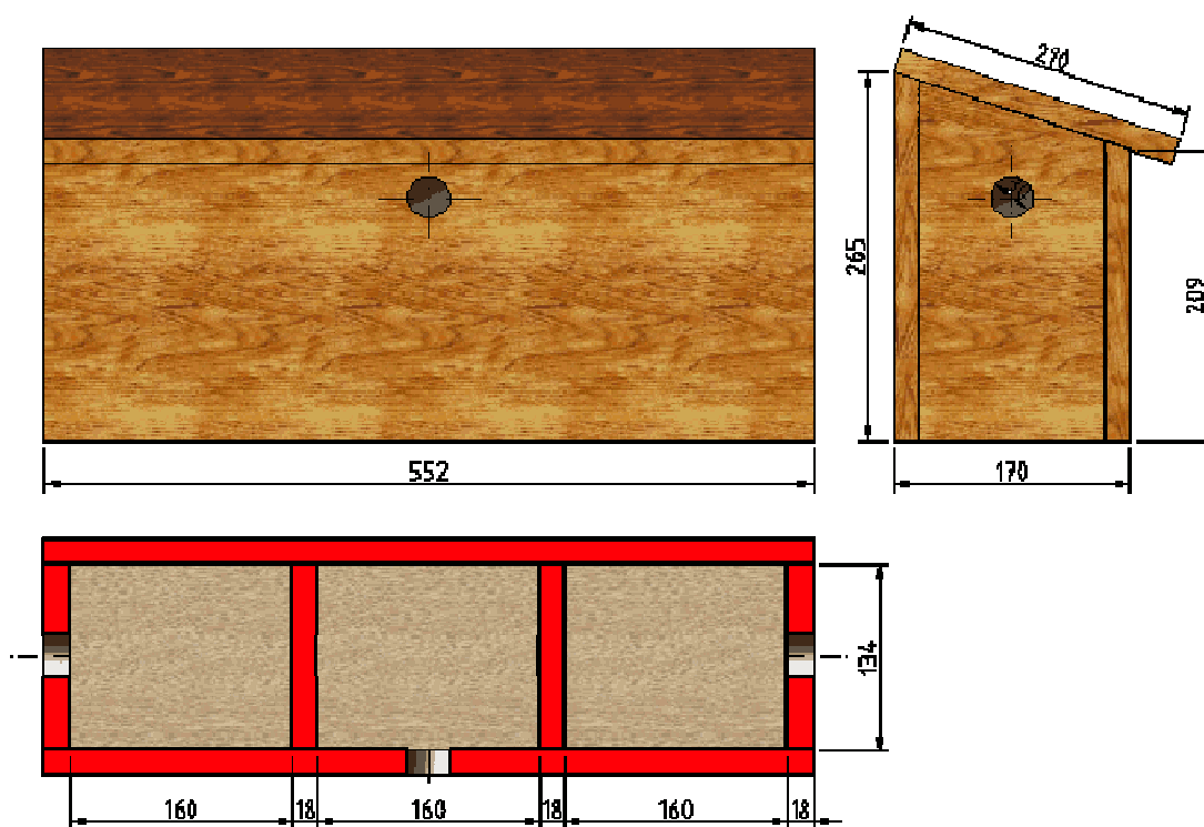
Figure 91 : Modèle de nichoir à Moineau domestique.
