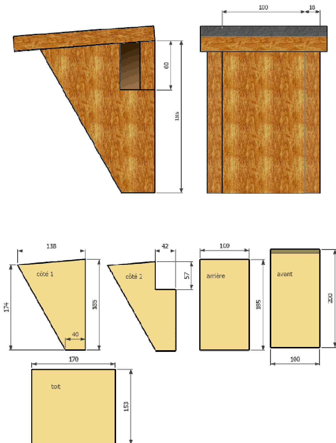
Figure 87 : Modèle de nichoir à Grimpereau.
